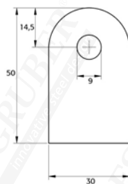
54306 Mat. 6 mm
