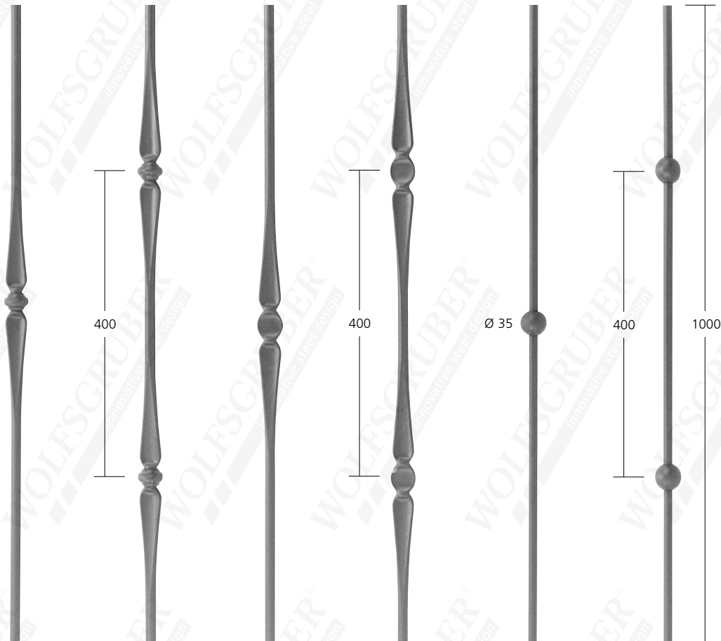
14200 Ø 12 0,93 kg 14202 Ø 14 1,28 kg
