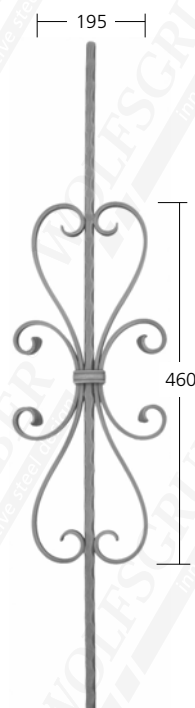
12545 ∅12 mm 2,00 kg
