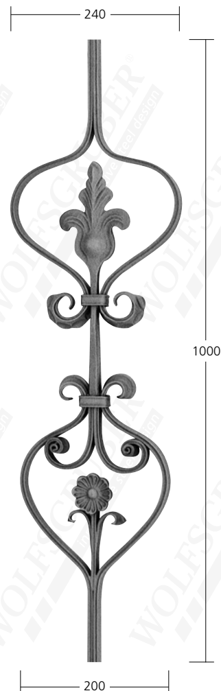
36980 Mat. 16x8 mm 3,60 kg
