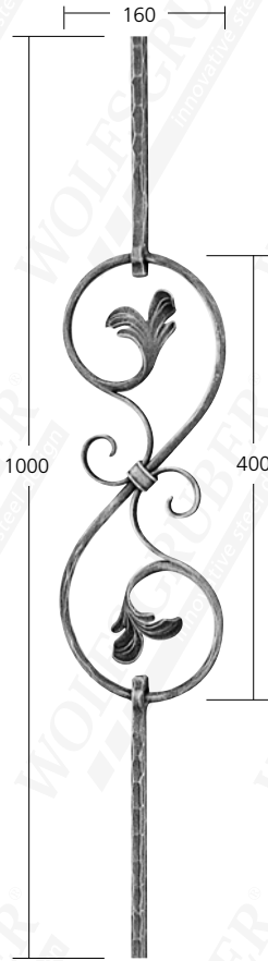
12104 ∅ 14 mm 1,48 kg
