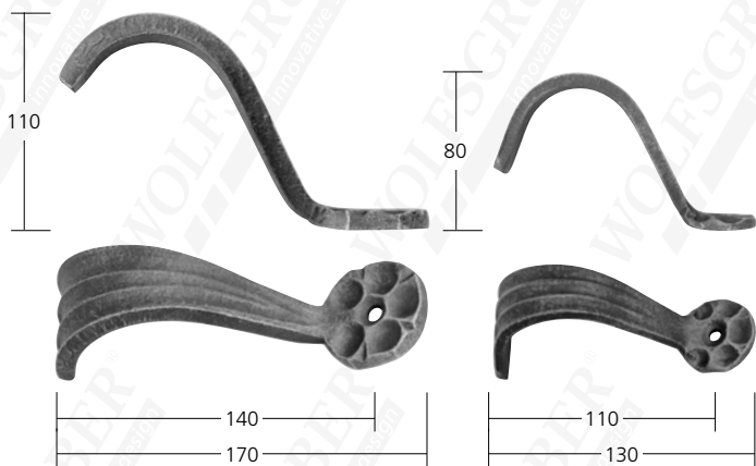
48010 Mat. 10 mm 0,50 kg
