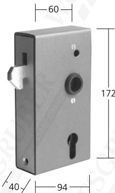
51460 1,78 kg
