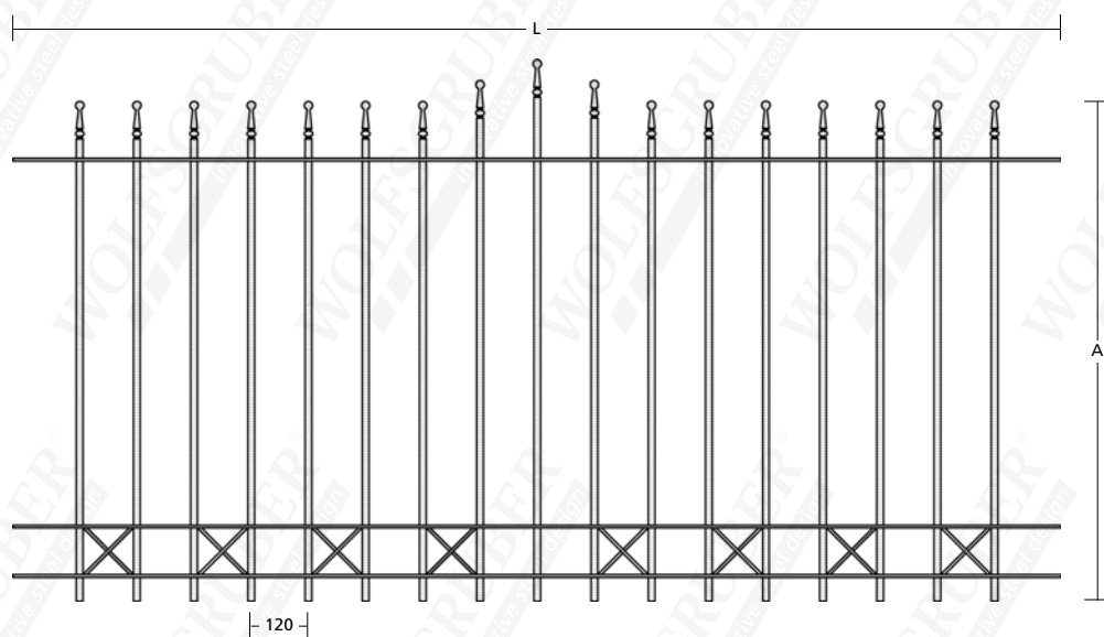
17608 25x8 | \varnothing 12mm - L: 2200 - A: 700
