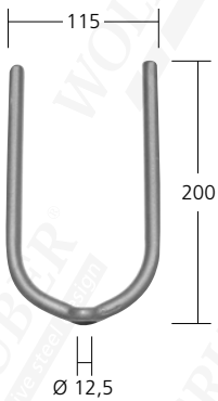
46115 Mat. Ø 12 mm 0,40 kg
