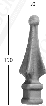
41318N Ø 41 mm 1,13 kg
