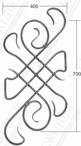
37052 Ø 12 mm
