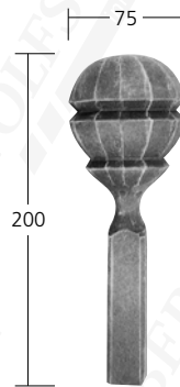
44010 ∅25 mm 2,46 kg
