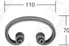
36462 Mat. 16x8 mm 0,34 kg
