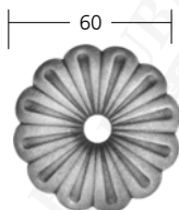
40060 Mat. 3 mm
