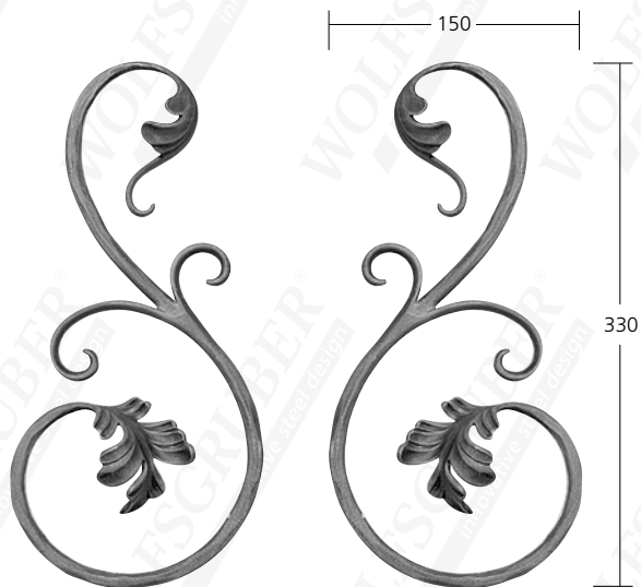
31210 Mat. Ø 10 mm 31211 0,54 kg
