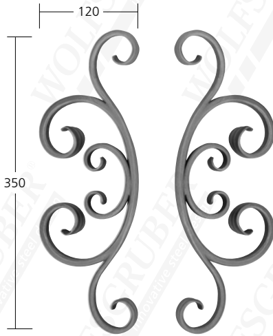
32430 Mat. 16x8 mm 0,95 kg
