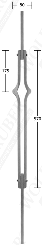
17140 \varnothing 12 mm
