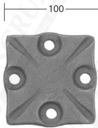
40632 Mat. 8 mm 0,40 kg
