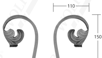
32210 Mat. 16x8 mm 32211 0,34 kg
