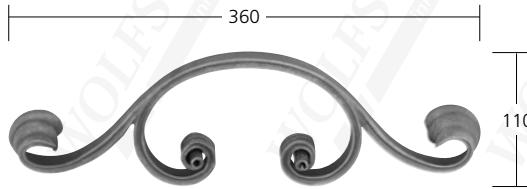
36450 Mat. 16x8 mm 0,80 kg
