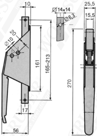
53120 0,90 kg
