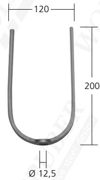
46135 Mat. 14x6 mm 0,31 kg
