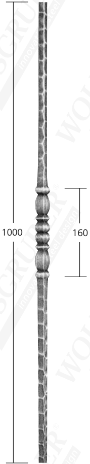
12416 \varnothing 14 mm 1,50 kg
