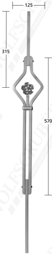
17112 \varnothing 12 mm
