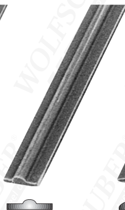
28318 18x5x2000 mm 28319 18x5x4000 mm 0,51 kg/m
