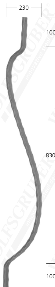
18252 Mat. 20x12 mm 2,15 kg
