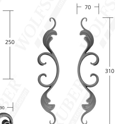
31824 Mat. Ø 10 mm 0,25 kg
