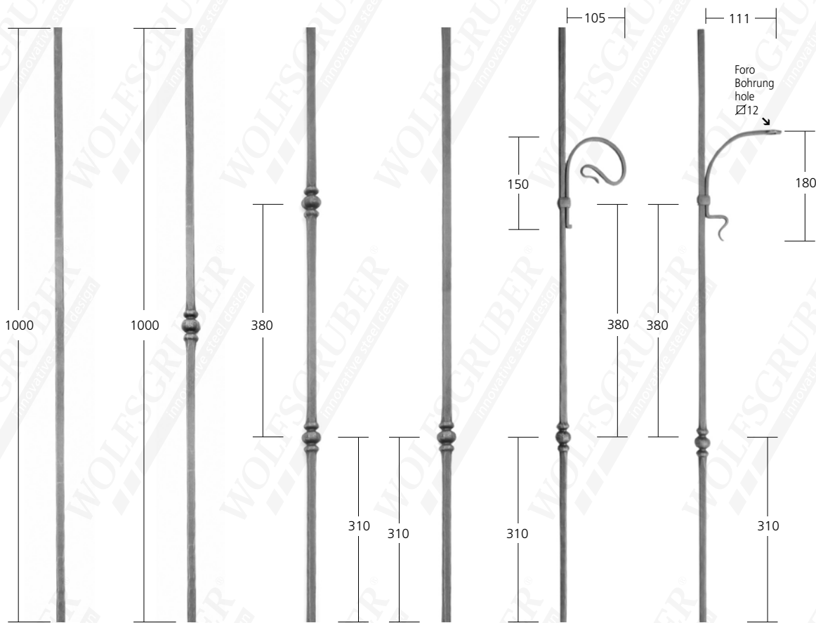
12464 Ø12 mm 1,00 kg
