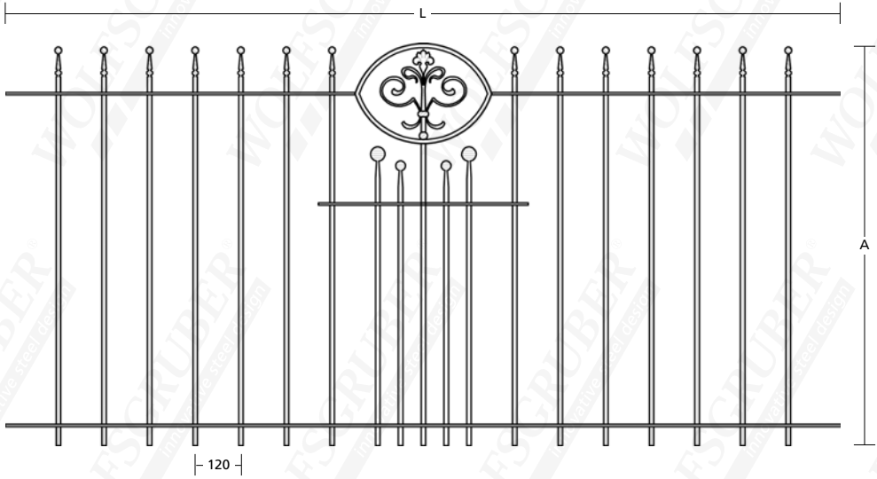
17600 25x8 l ø 12mm - L: 2200 - A: 700
