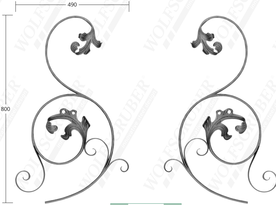
31018 Mat. Ø 12 mm 31019 2,60 kg
