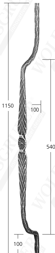
18020 \varnothing 12 mm 1,25 kg
