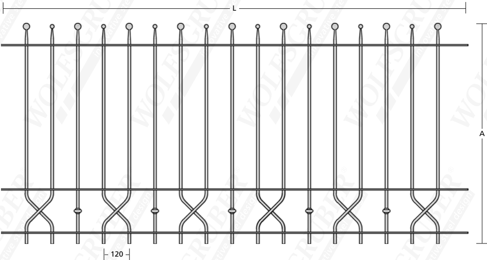
17623 25x8 l ø 12mm - L: 2200 - A: 700
