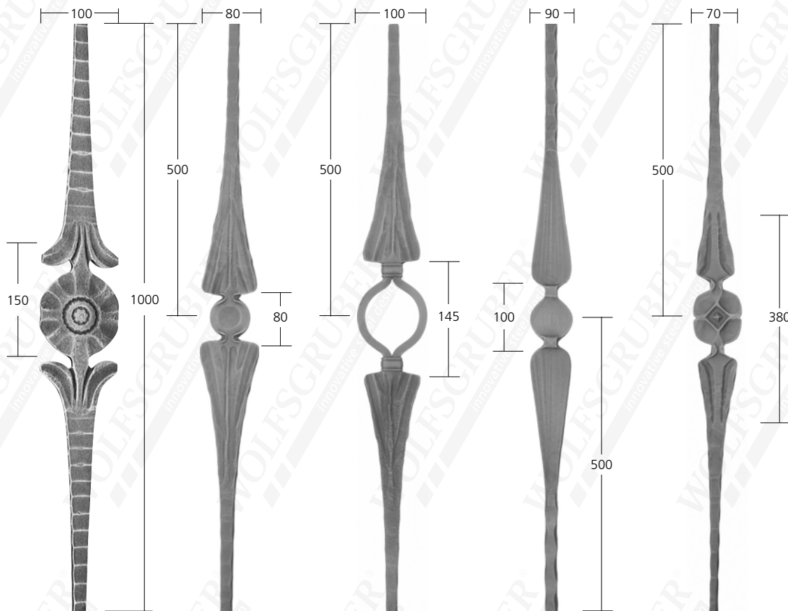
12316 Mat. 8x18 mm 2,52 kg
