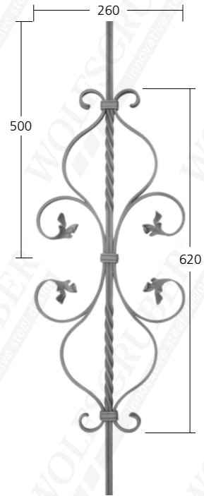
12622 12 mm 2,10 kg
