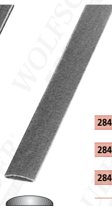
28116 16x4x3000 mm 0,46 kg/m
