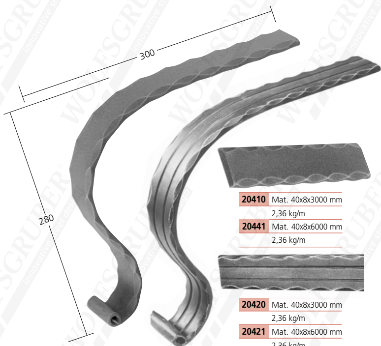
20412 Mat. 40x8 mm 1,42 kg
