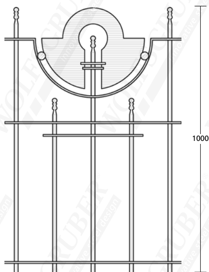
17510-E
