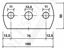
45200 0,21 kg
