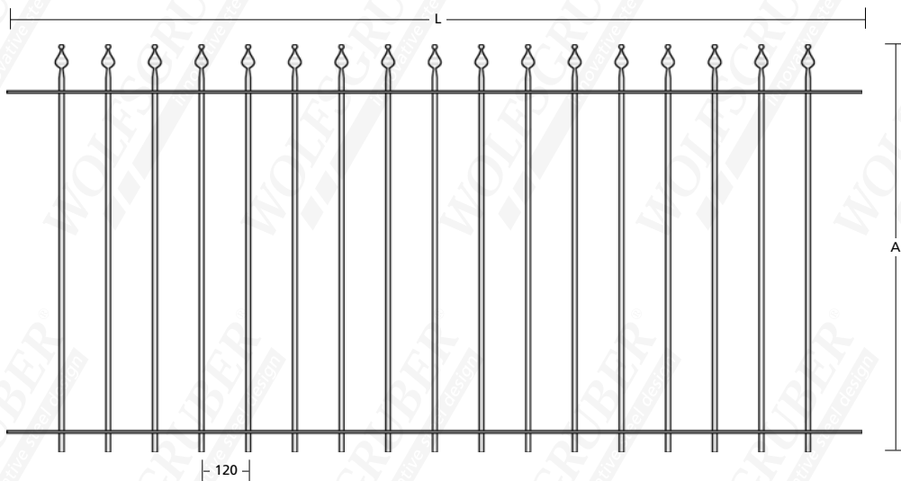
17618 25x8 | \varnothing 12mm - L: 2200 - A: 700
