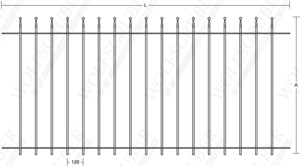
17603 25x8 l ø 12mm - L: 2200 - A: 700
