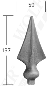
41414 \varnothing 14 mm 0,30 kg
