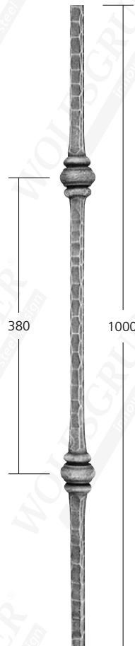
12413 \varnothing 14 mm 2,50 kg
