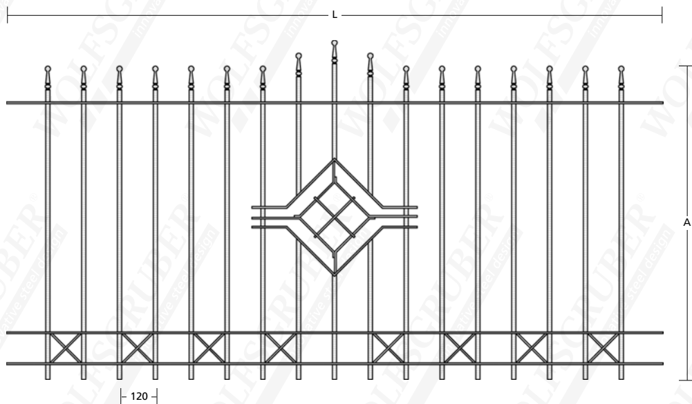
17605 25x8 | \varnothing 12mm - L: 2200 - A: 700
