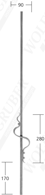
17090 \varnothing 12 mm 1,38 kg
