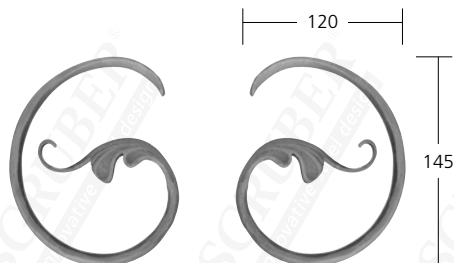
31250 Mat. Ø 10 mm 31251 0,22 kg
