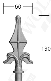
41360 Ø 11 mm 0,17 kg
