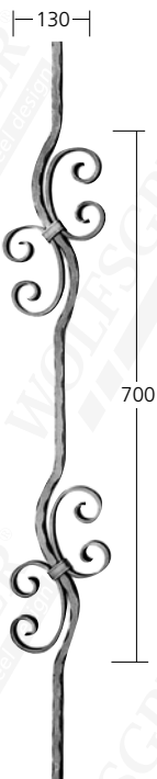
12568 ∅12 mm 1,80 kg
