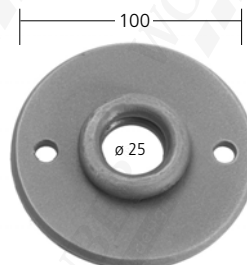
40622 Mat. 6 mm 0,34 kg
