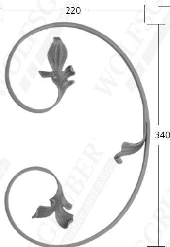
36151 Mat. 12x5 mm 0,54 kg
