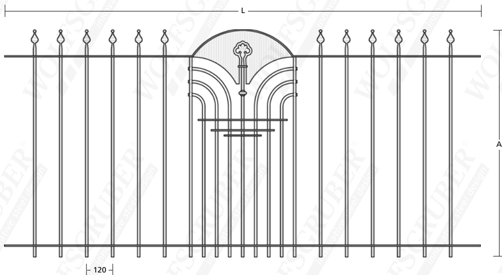
17615 25x8 | \varnothing 12mm - L: 2200 - A: 700
