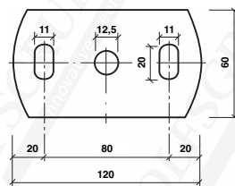
45220 0,28 kg
