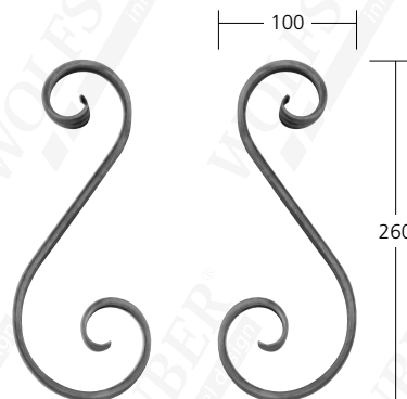
32462 Mat. 16x8 mm 0,70 kg
