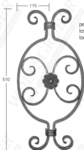
31950 Mat. 14x6-8 mm 2,40 kg
