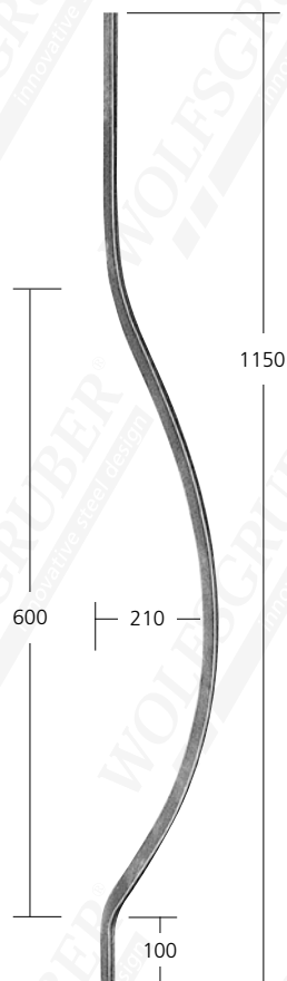
18112 16x8 mm 1,14 kg
