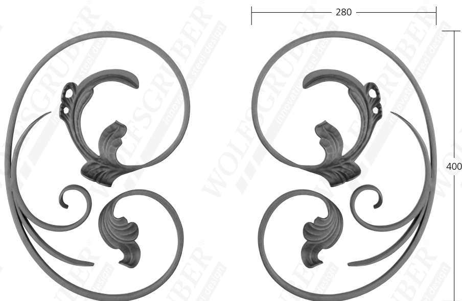
32250 Mat. 16x8 mm 32251 1,84 kg
