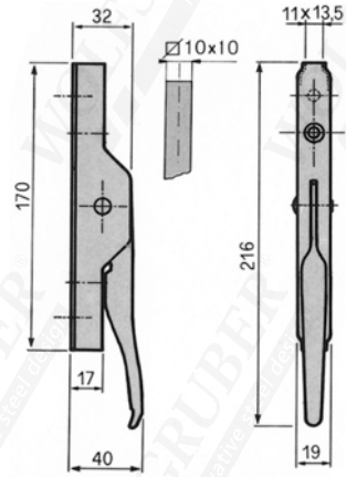
53130 0,50 kg
