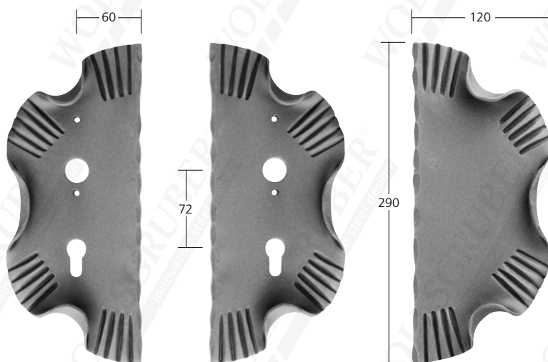
51120 Mat. 4 mm 0,70 kg
