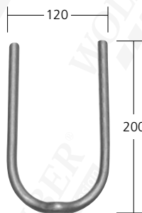
46125 Mat. Ø 12 mm 0,40 kg
