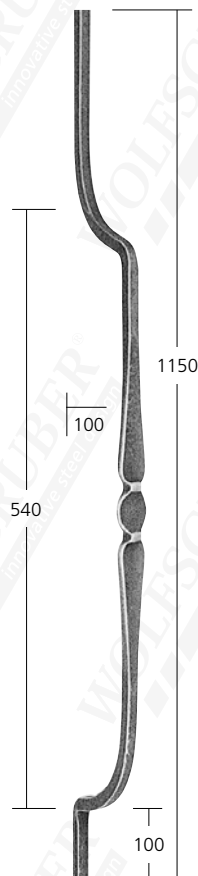
18008 Ø 14 mm 1,88 kg
